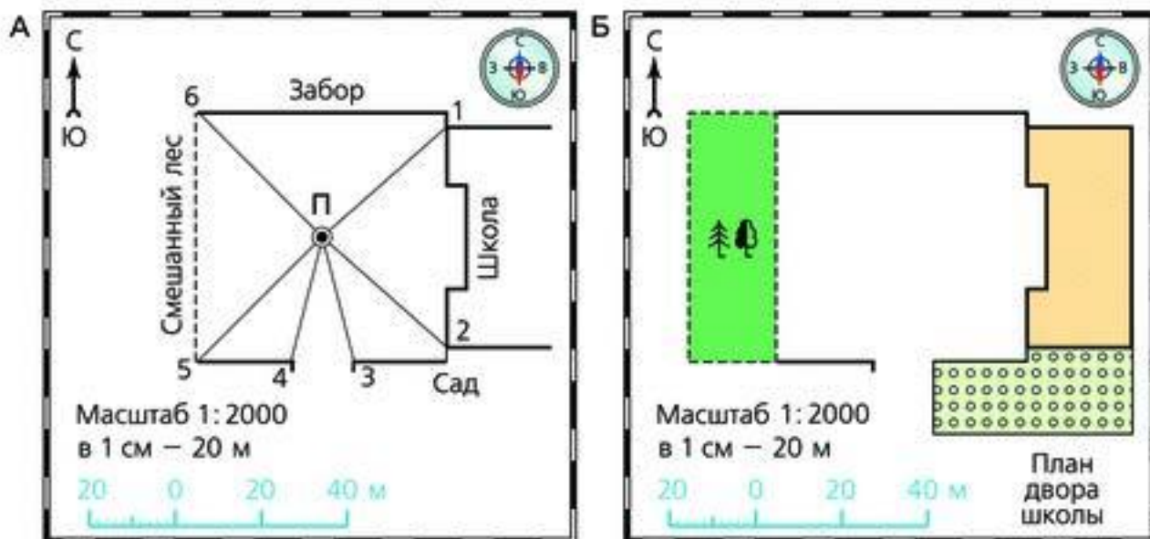
Рис. 16. Полярная съёмка:
