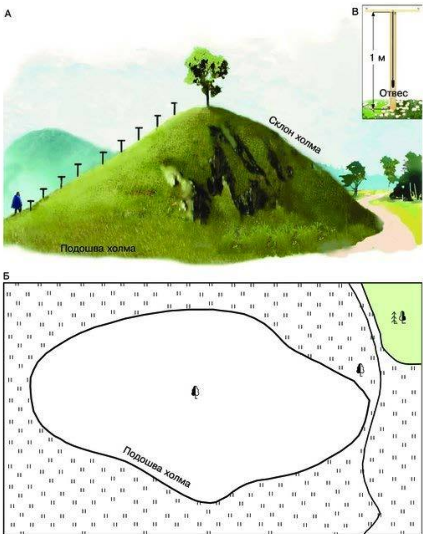
Рис. 10. А — общий вид холма; Б — план местности с изображением подошвы холма; В — самодельный нивелир
