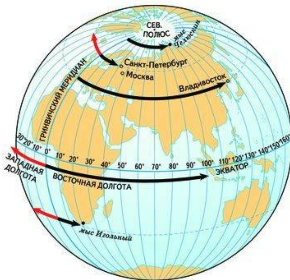
Рис. 22. Географическая долгота
