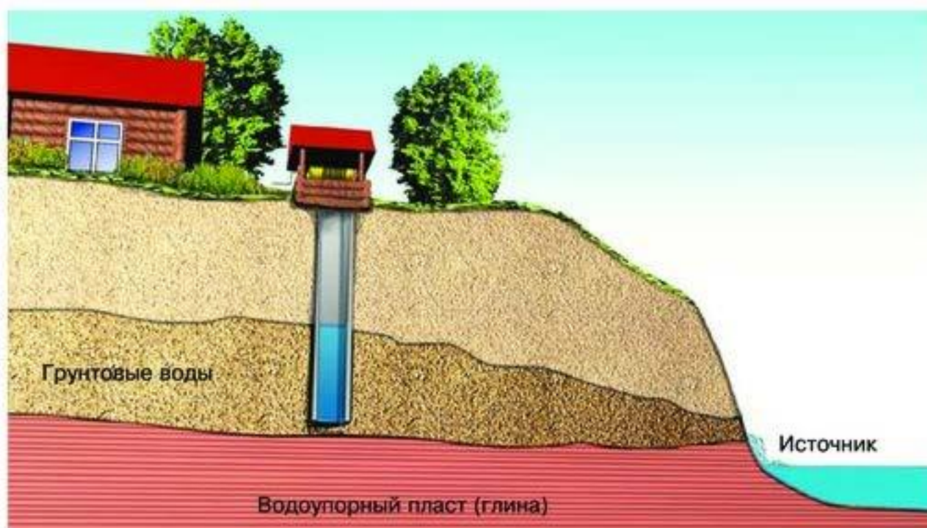
Рис. 56. Грунтовые воды
