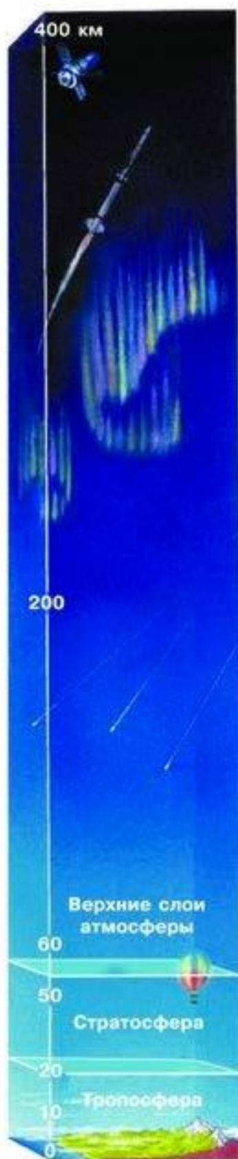
Рис. 68. Строение атмосферы
