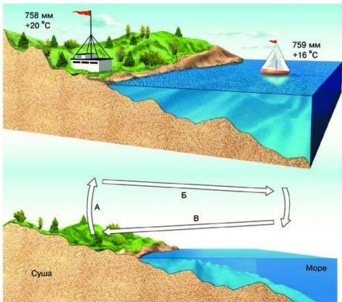
Рис. 74. Дневной бриз
