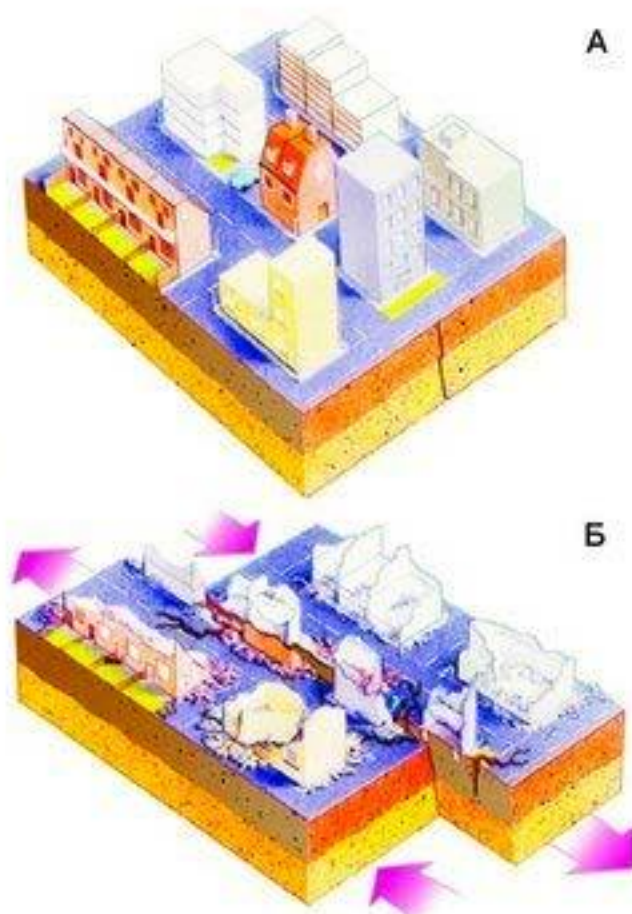
Рис. 29. После землетрясения
