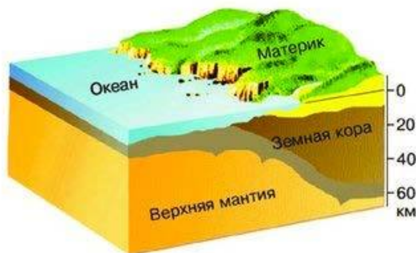
Рис. 25. Литосфера
