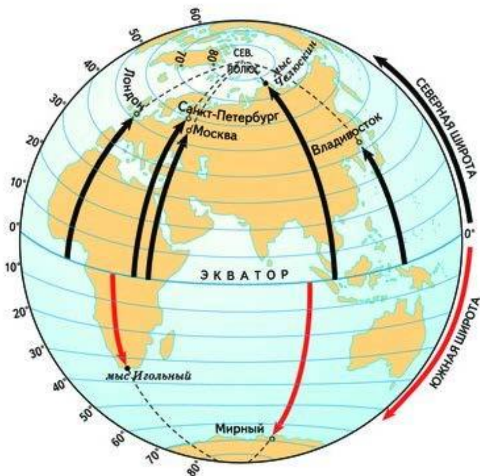
Рис. 20. Географическая широта
