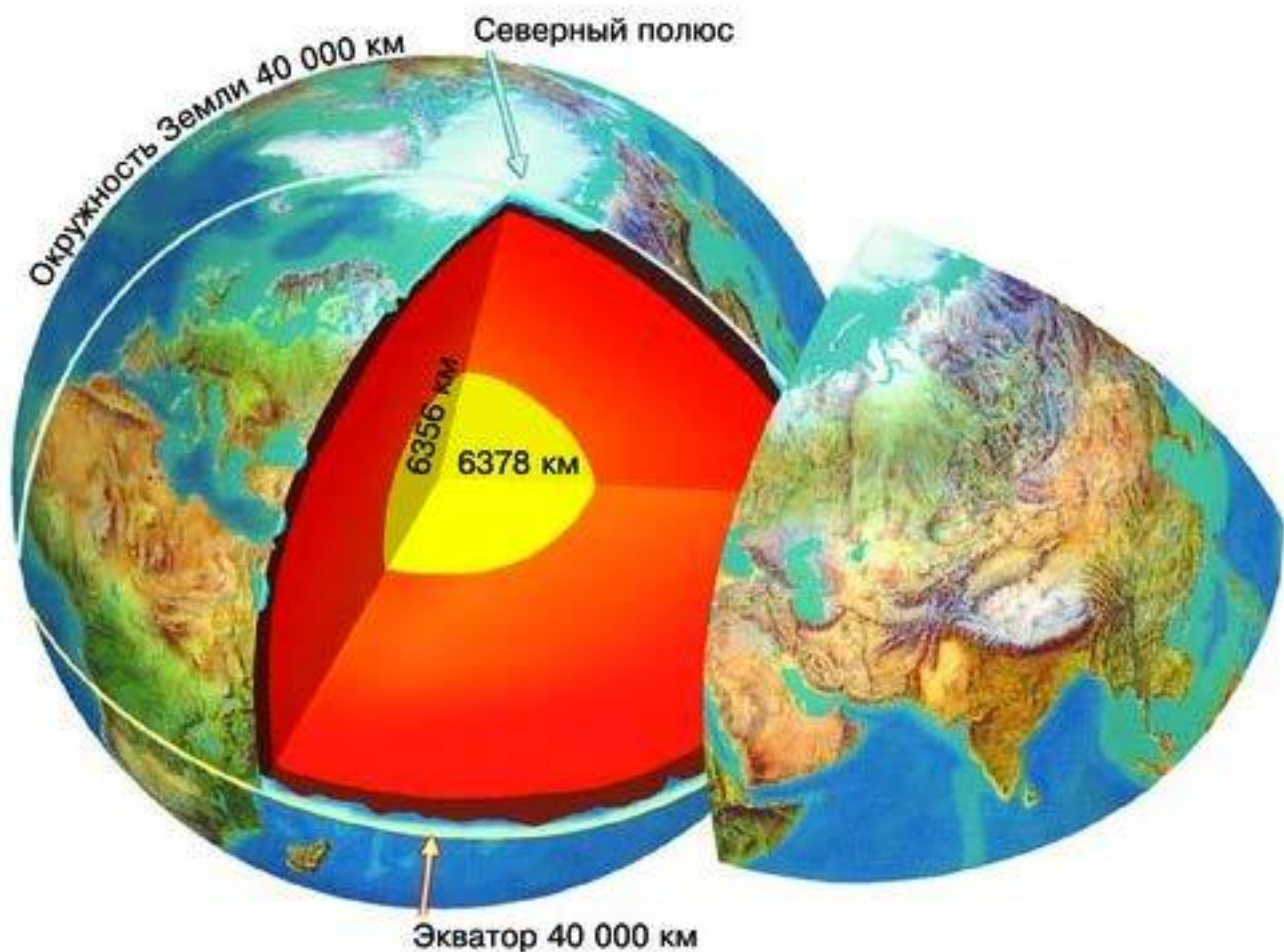
Рис. 18. Размеры Земли
