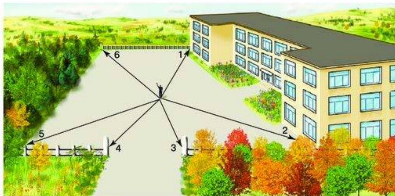
Рис. 15. Полярная съёмка: общий вид участка
